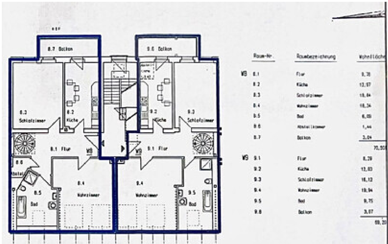
Grundriss unten
